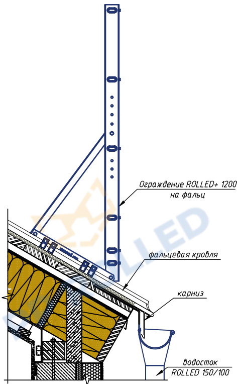
Типовой узел крепления ограждения на фальцевую кровлю
