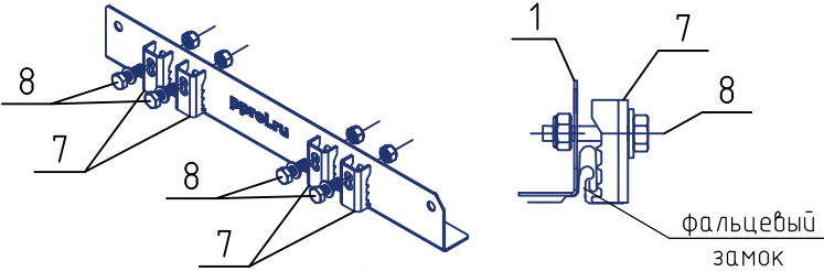
Опора РП-ОГ в сборе
