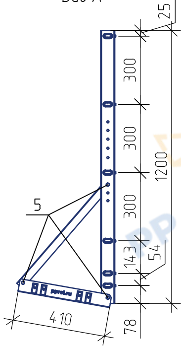
Вид А
