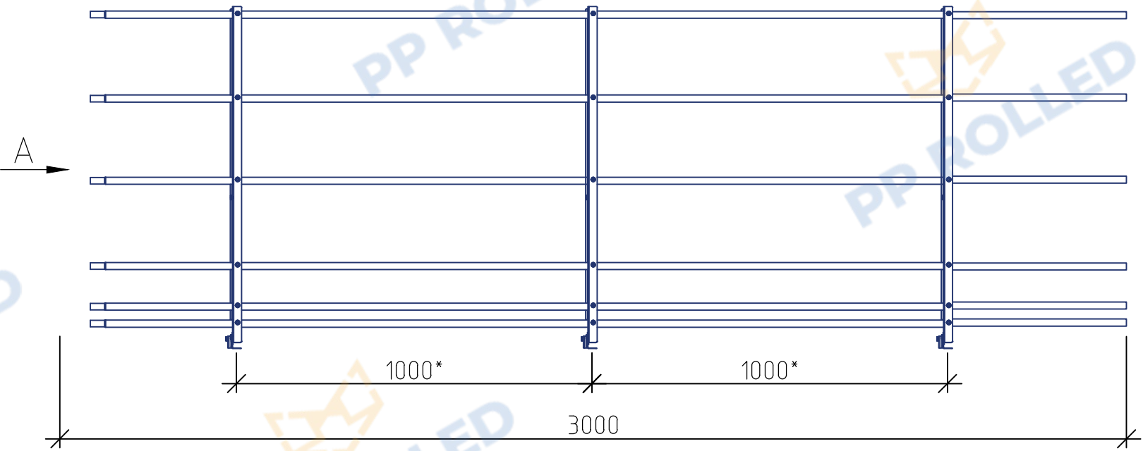
Ограждение РПФ-ОГ-1200 (l=3000мм) + ФС PP ROLLED
