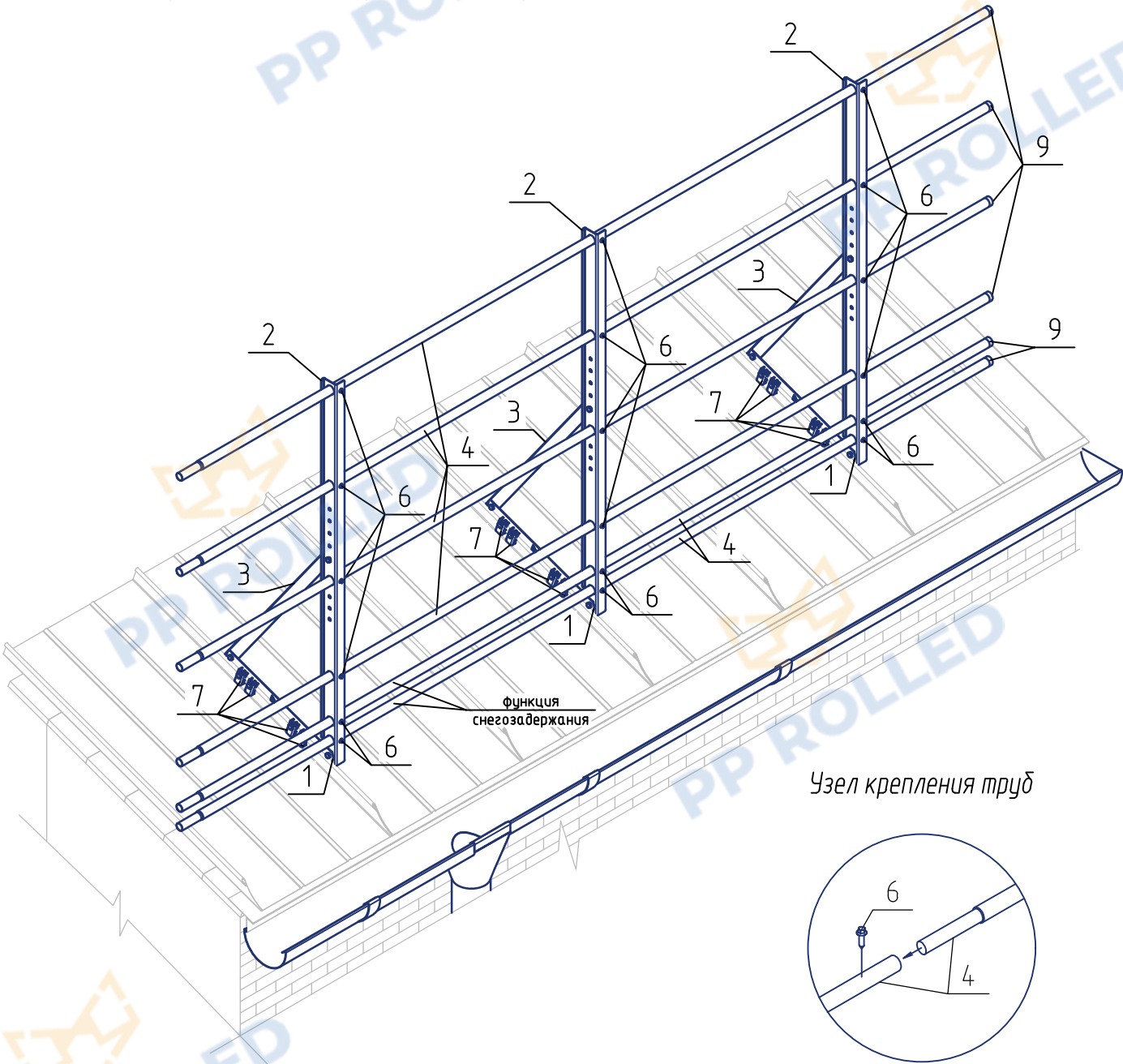
Типовой узел крепления ограждения на фальцевую кровлю
