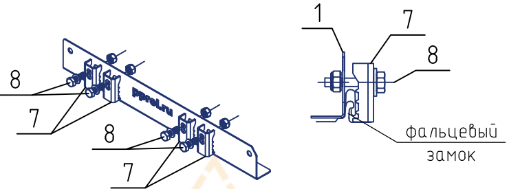
Опора РП-ОГ в сборе
