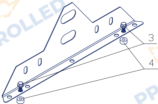
Опора РП-СН-40х20
