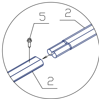
Узел крепления труб
