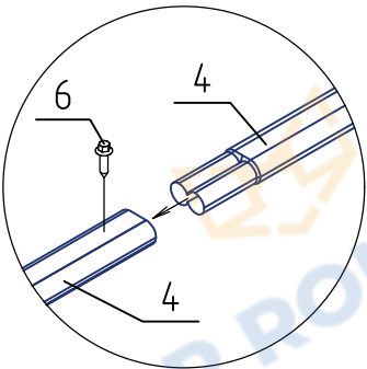
Узел крепления трубы
