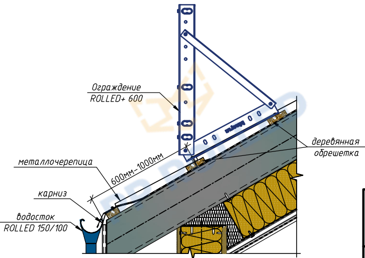
Типовой узел крепления ограждения на металлочерепицу
