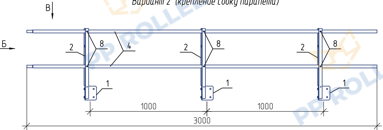
Ограждение РП-ПРС-600 (L=3000 мм) PP ROLLED Вариант 2 (крепление сбоку парапета)
