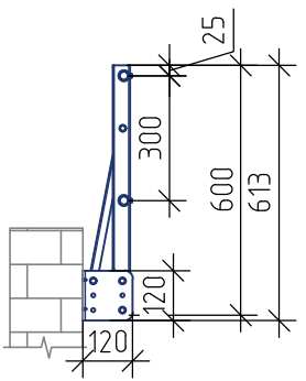
Вид Б
