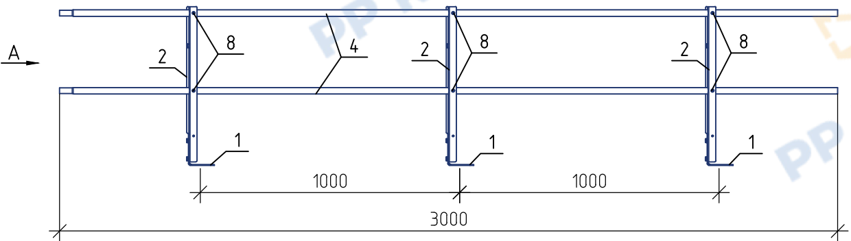
Ограждение РП-ПРС-600 (L=3000 мм) PP ROLLED Вариант 1 (крепление на парапет)
