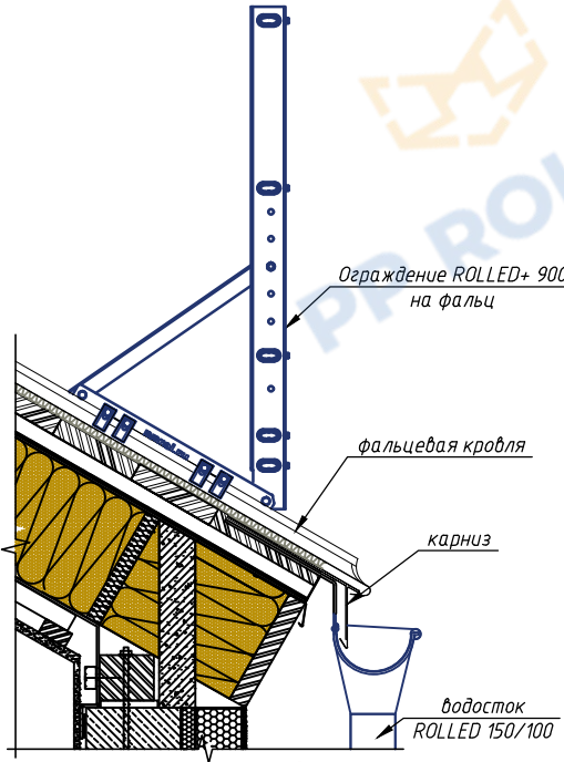
Сечение опорной стойки РП-ОГ-900
