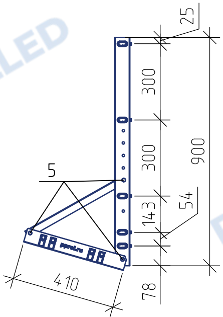
Типовой узел крепления ограждения на фальцевую кровлю
