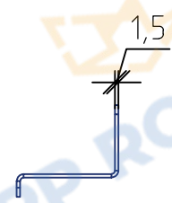
Сечение опорной стойки РП-ОГ-600
