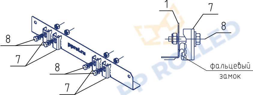
Опора РП-ОГ в сборе
