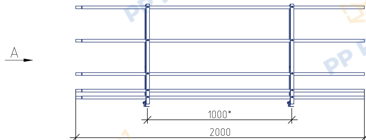
Ограждение РПФ-ОГ-900 (l=2000мм)+ФС PP ROLLED
