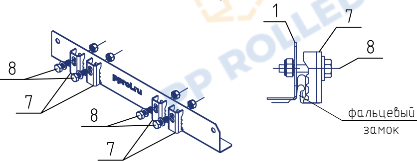
Опора РП-ОГ в сборе
