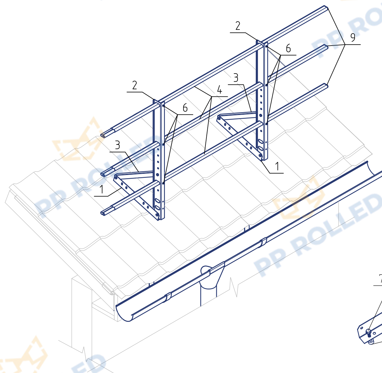
Узел крепления к кровле
