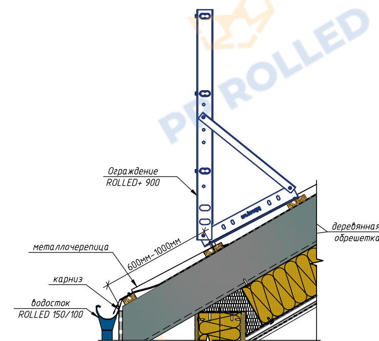
Типовой узел крепления ограждения на металлочерепицу
