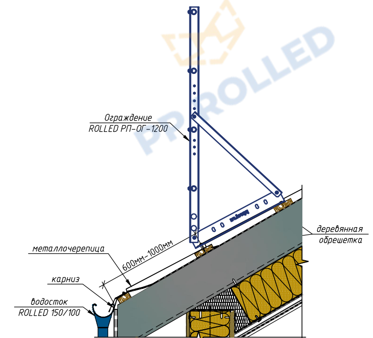
Типовой узел крепления ограждения на металлочерепицу
