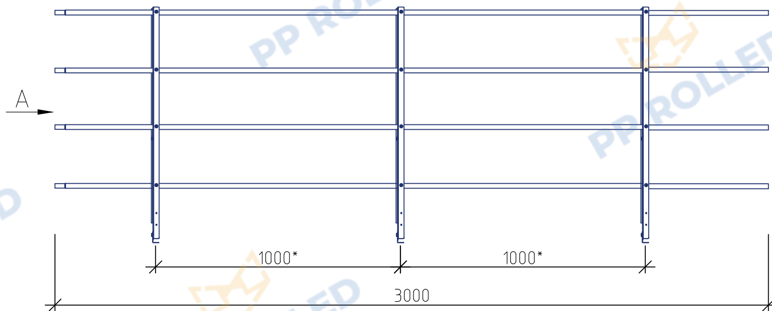
Ограждение РП-ОГ-1200 (l=3000мм) PP ROLLED
