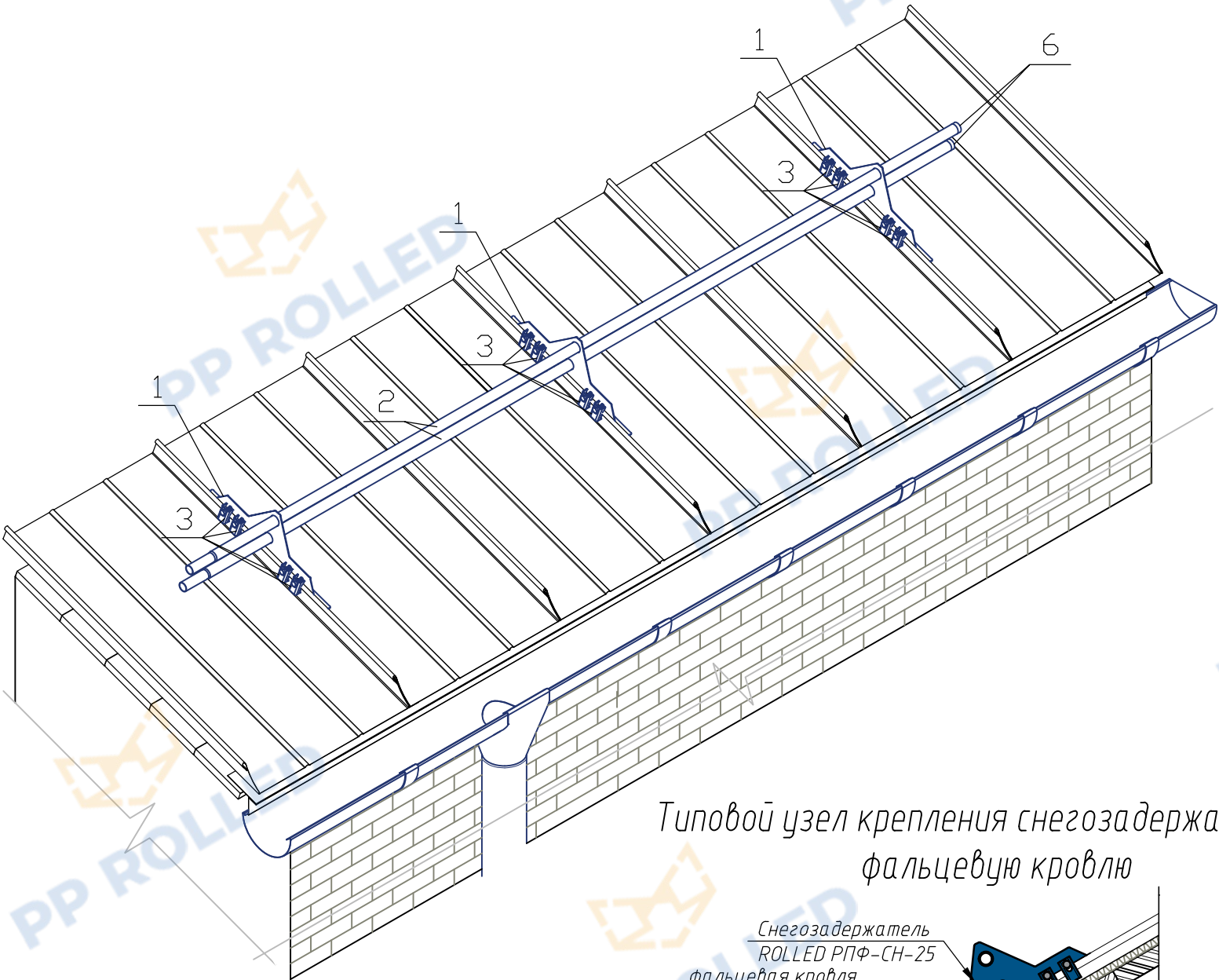
Узел крепления трубы
