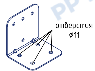
Опора РП-ДЕК-ПРС
