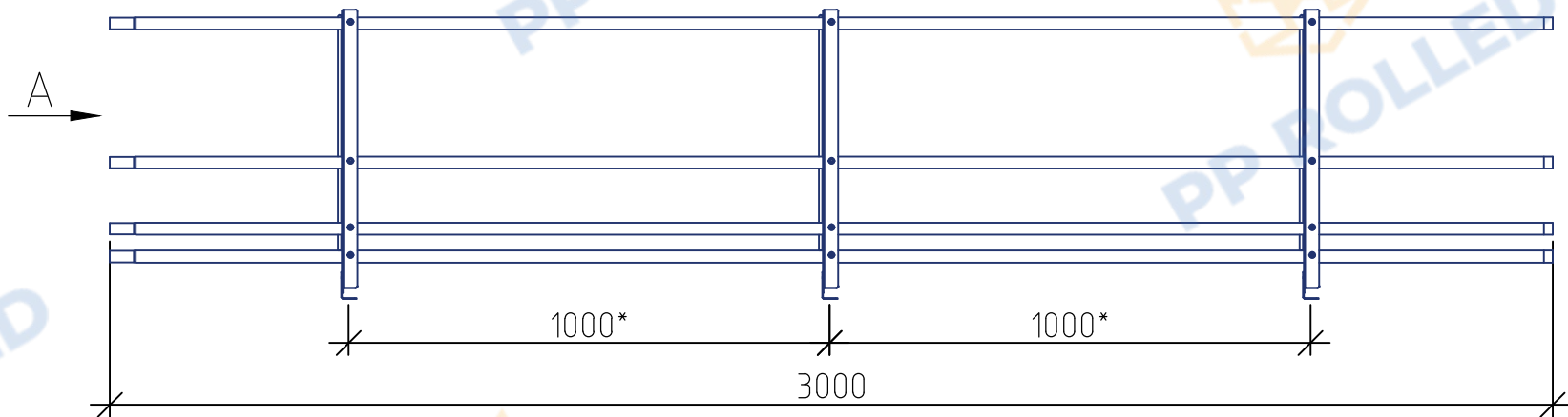
Ограждение РП-ОГ-600 (l=3000)+ФС PP ROLLED
