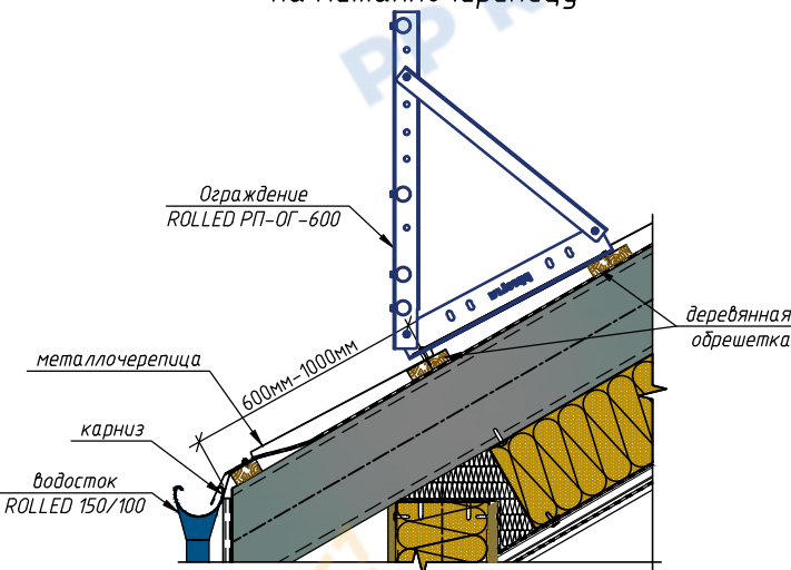
Типовой узел крепления ограждения на металлочерепицу
