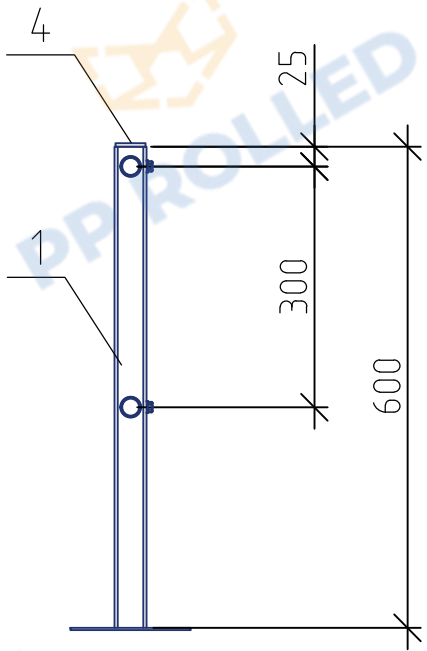
Вид А
