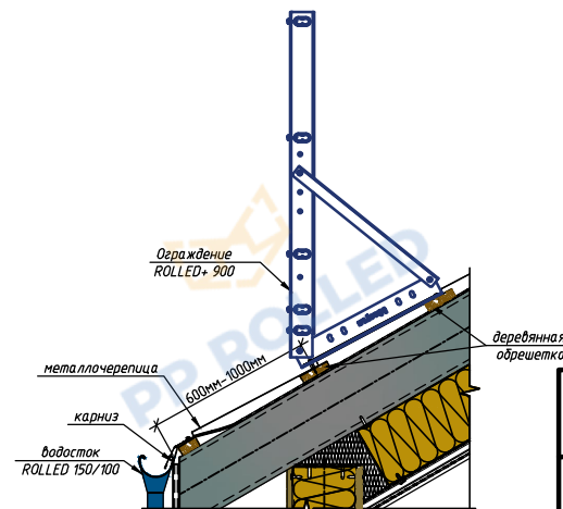
Типовой узел крепления ограждения на металлочерепицу
