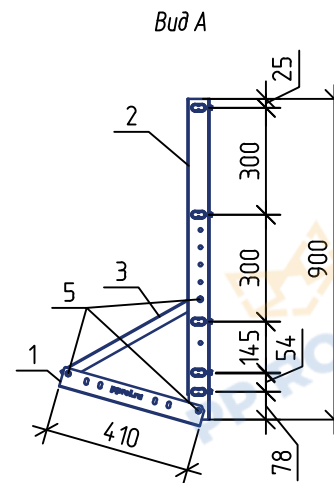
Узел крепления труб
