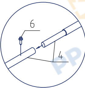
Узел крепления труб
