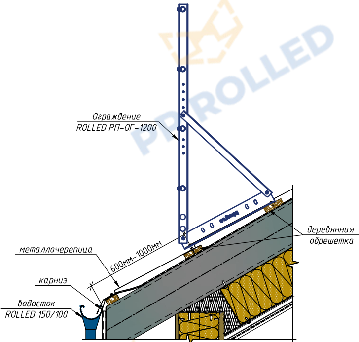
Типовой узел крепления ограждения на металлочерепицу
