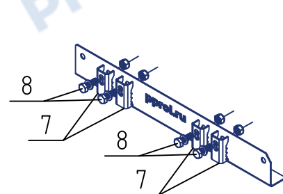
Опора РП-ОГ в сборе
