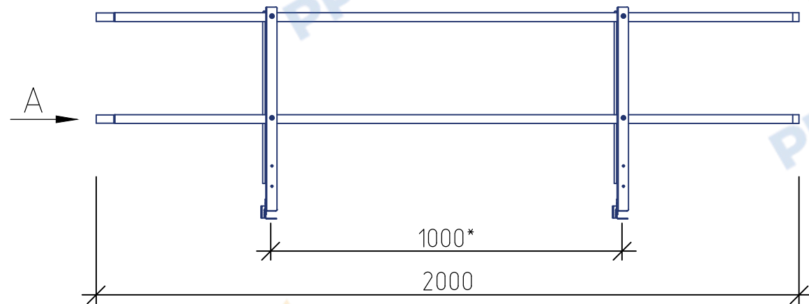
Ограждение РПФ-ОГ-600 (l=2000мм) PP ROLLED
