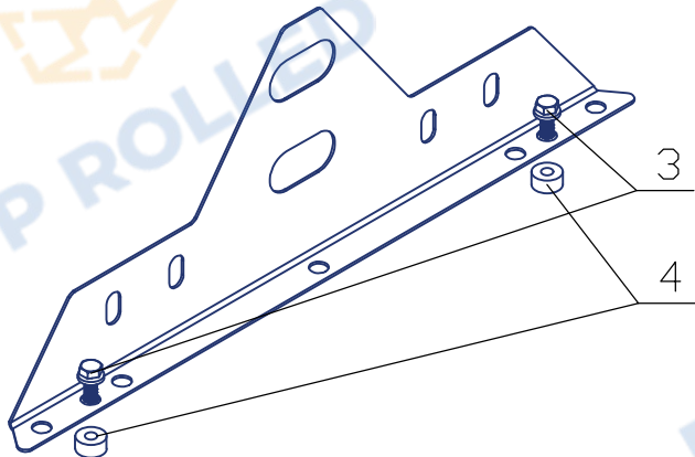
Опора РП-СН-40х20
