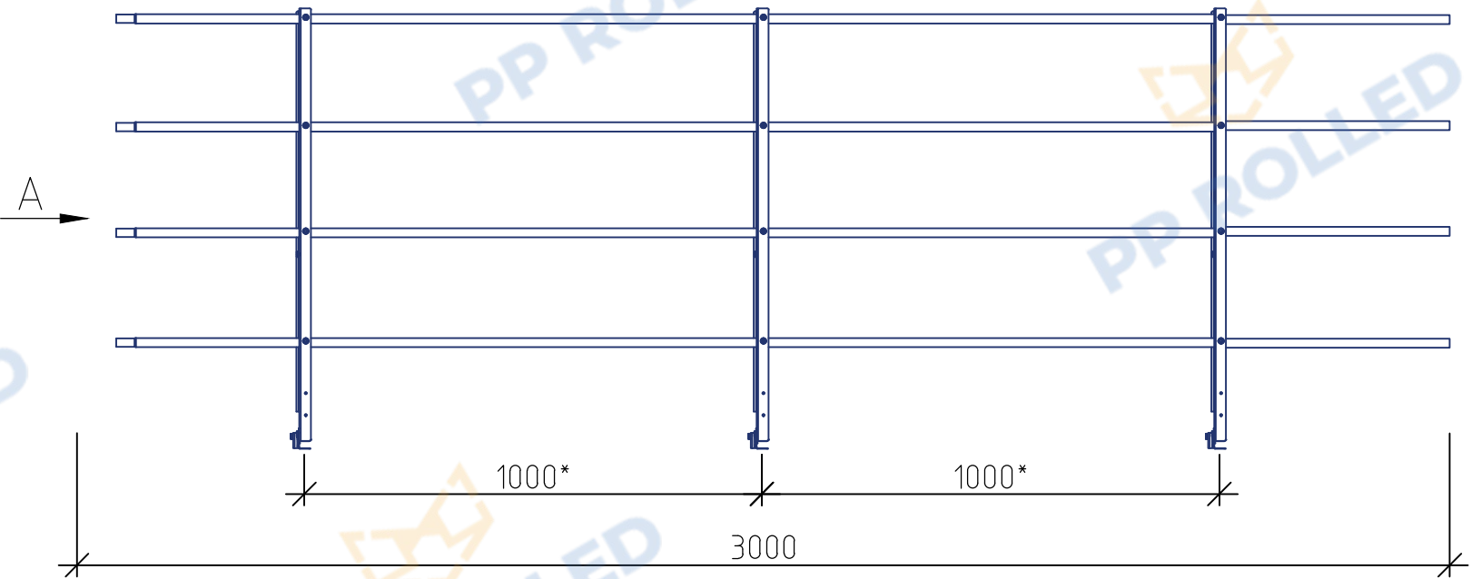
Ограждение РПФ-ОГ-1200 (l=3000мм) PP ROLLED
