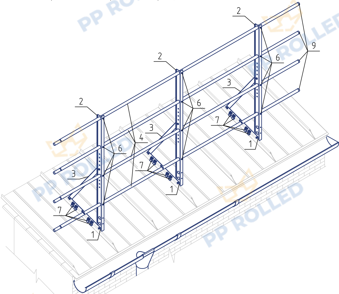
Типовой узел крепления ограждения на фальцевую кровлю
