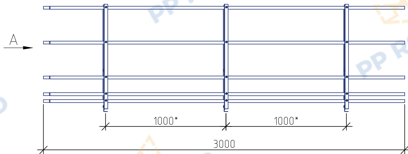
Ограждение РП-ОГ-900 (L=3000мм)+ФС PP ROLLED
