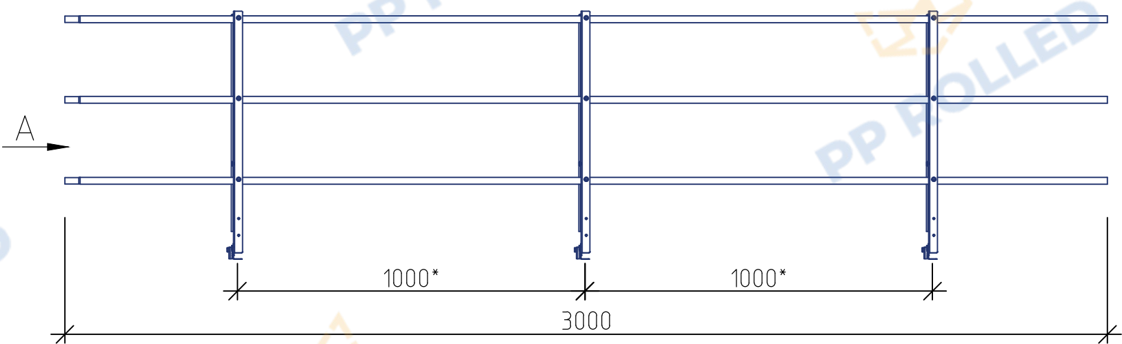
Ограждение РПФ-ОГ-900 (l=3000мм) PP ROLLED
