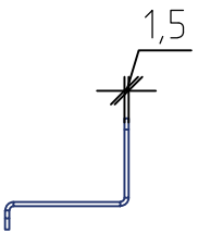
Сечение опорной стойки РП-ОГ-600
