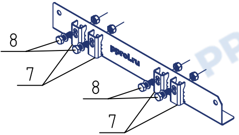
Опора РП-ОГ в сборе
