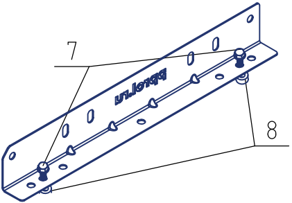
Узел крепления к кровле
