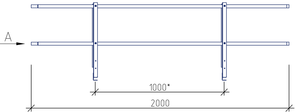
Ограждение РП-ОГ-600 (l=2000) PP ROLLED
