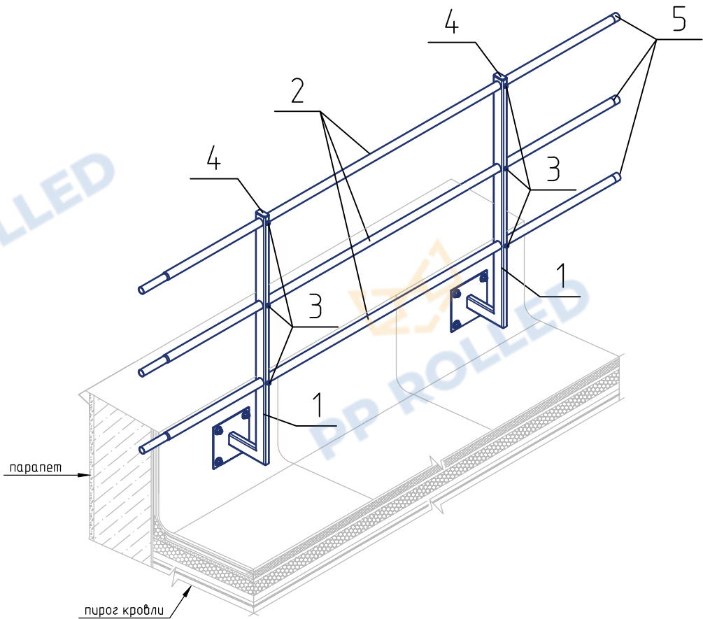
Ограждение РП-ОГ-ПР-У-900 (l=2000 мм)-ДТ (общий вид)
