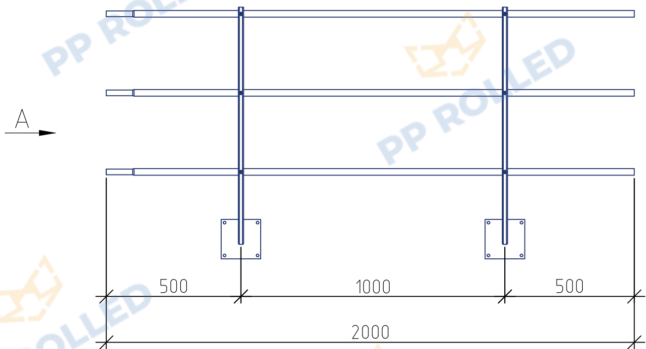
Ограждение РП-ОГ-ПР-У-900 (l=2000 мм) PP ROLLED
