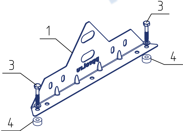
Крепление опоры
