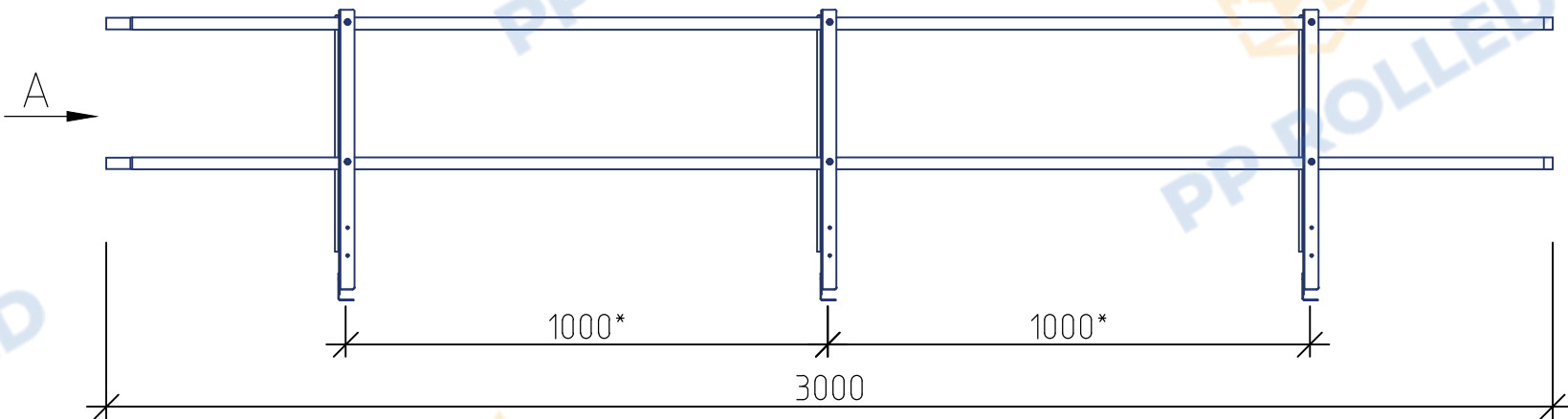
Ограждение РП-ОГ-600 (l=3000) PP ROLLED
