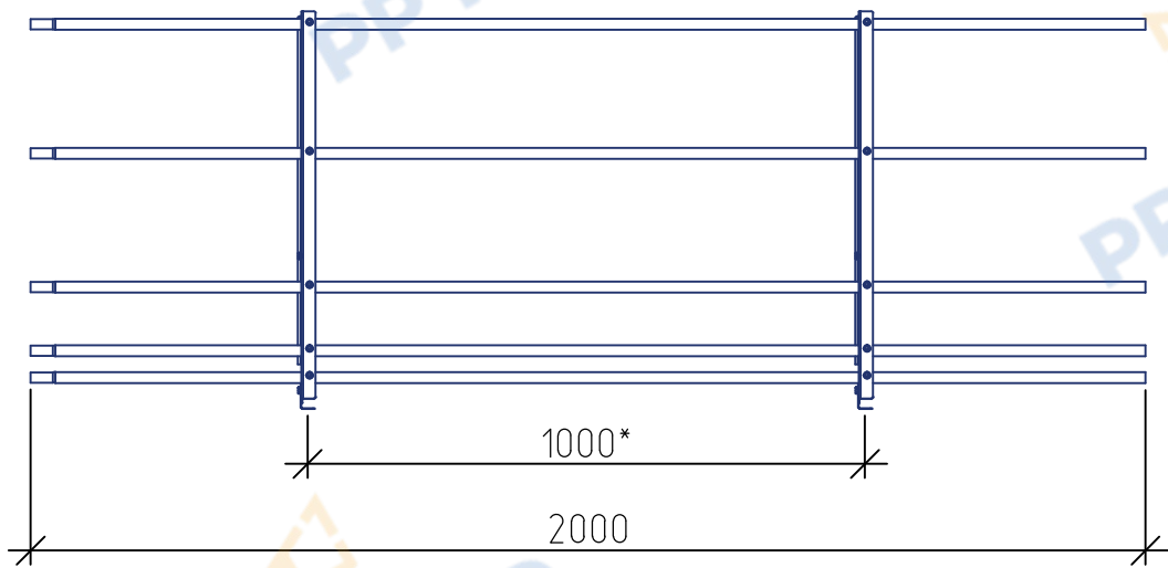
Ограждение РП-ОГ-900 (L=2000мм)+ФС PP ROLLED
