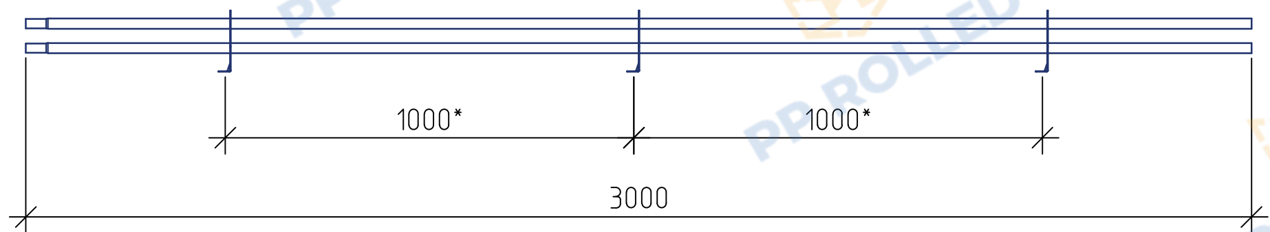
Снегозадержатель ROLLED+ 25-1.5 L=3000мм (3 опоры) PP ROLLED
