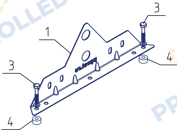
Крепление опоры
