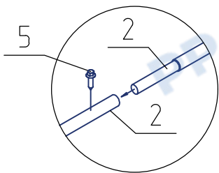
Узел крепления труб
