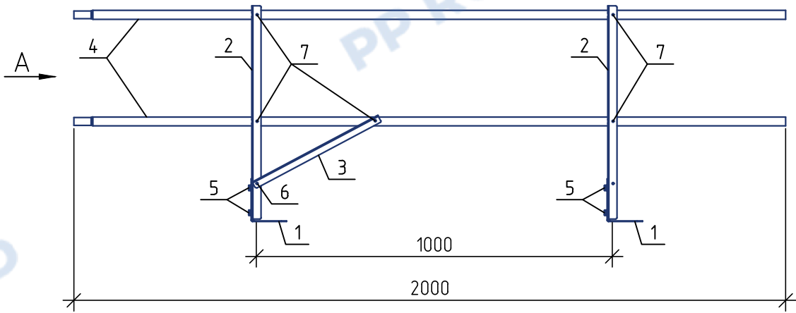
Ограждение РП-ДЕК-ПРС-600 (l=2000 мм) PP ROLLED Вариант 2 (крепление сбоку парапета)
