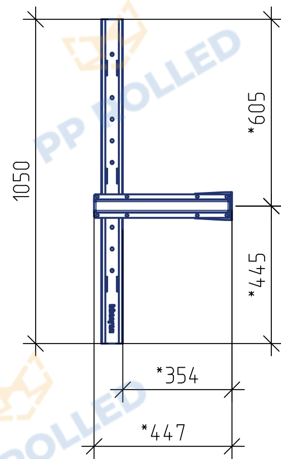
Вид А
