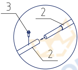
Узел крепления труб
