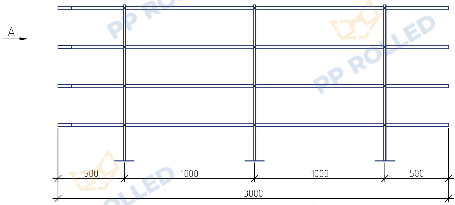
Ограждение РП-ОГ-ПР-1200 (l=3000 мм) -2ДТ (общий вид)
