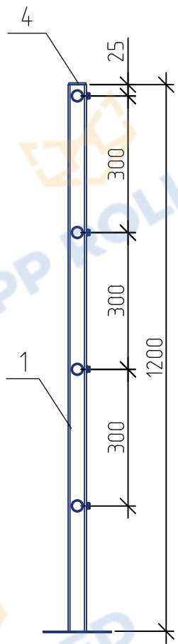
Вид А
